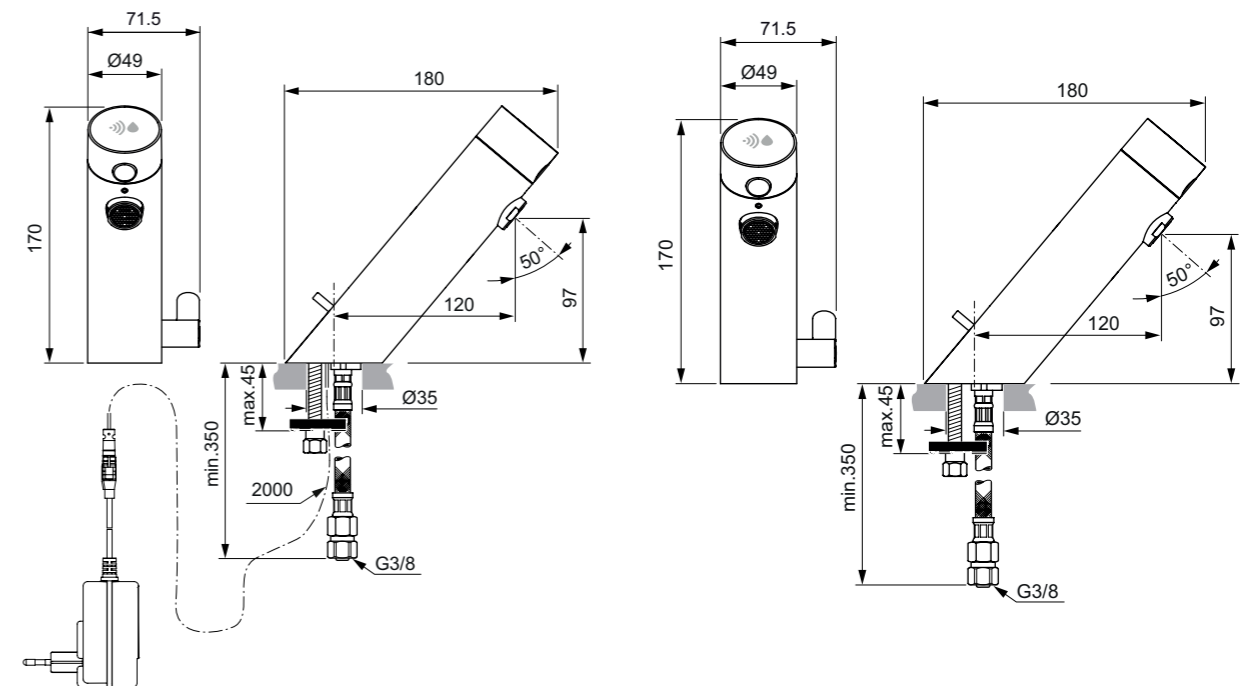
A7558
