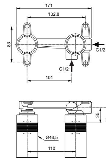
A1313
