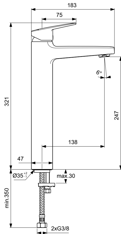
BD236
